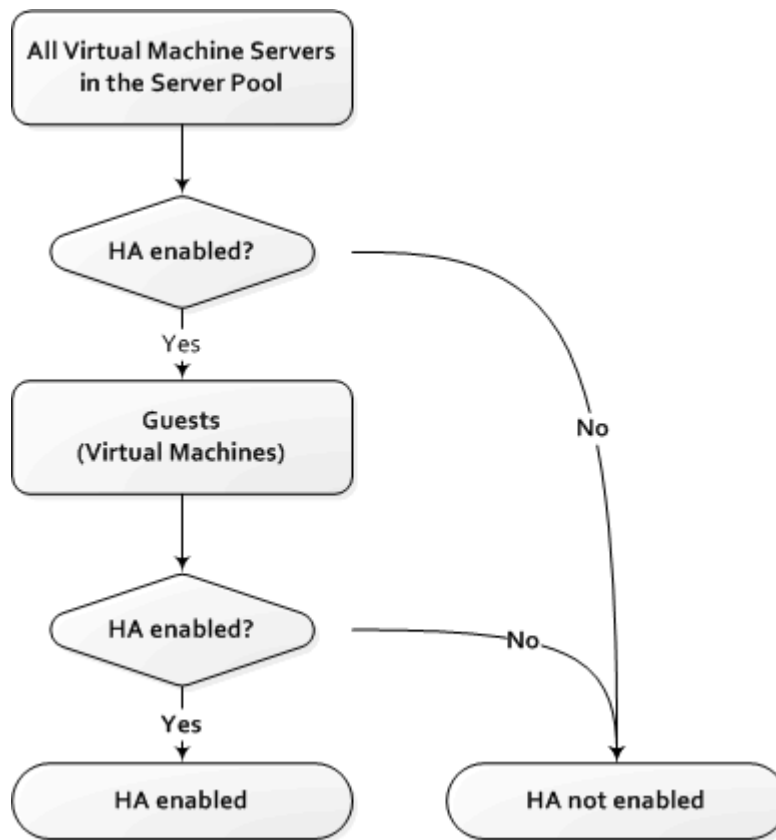
Figure 4: Oracle VM HA Checklist
